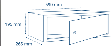
Dimensions du coffre intérieur
